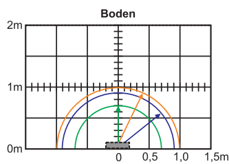
Lampenlichtstrom Not (DC) / Netz: 80lm
